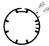
Item No.: GL1153 W: 1.43kg/m T: 2.0mm OD: \Phi 62mm ID: \Phi 58mm
