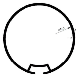
Item No.: GL1081 W: 0.71kg/m T: 1.6mm OD: \Phi 50.3mm ID: \Phi 47.1mm
