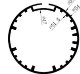
Item No.: GL1009 W: 1.02kg/m T: 1.5mm OD: \Phi 57.3mm ID: \Phi 54.3mm
