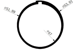
Item No.: GL1094 W: 1.0kg/m T: 1.5mm OD: \Phi 47mm
